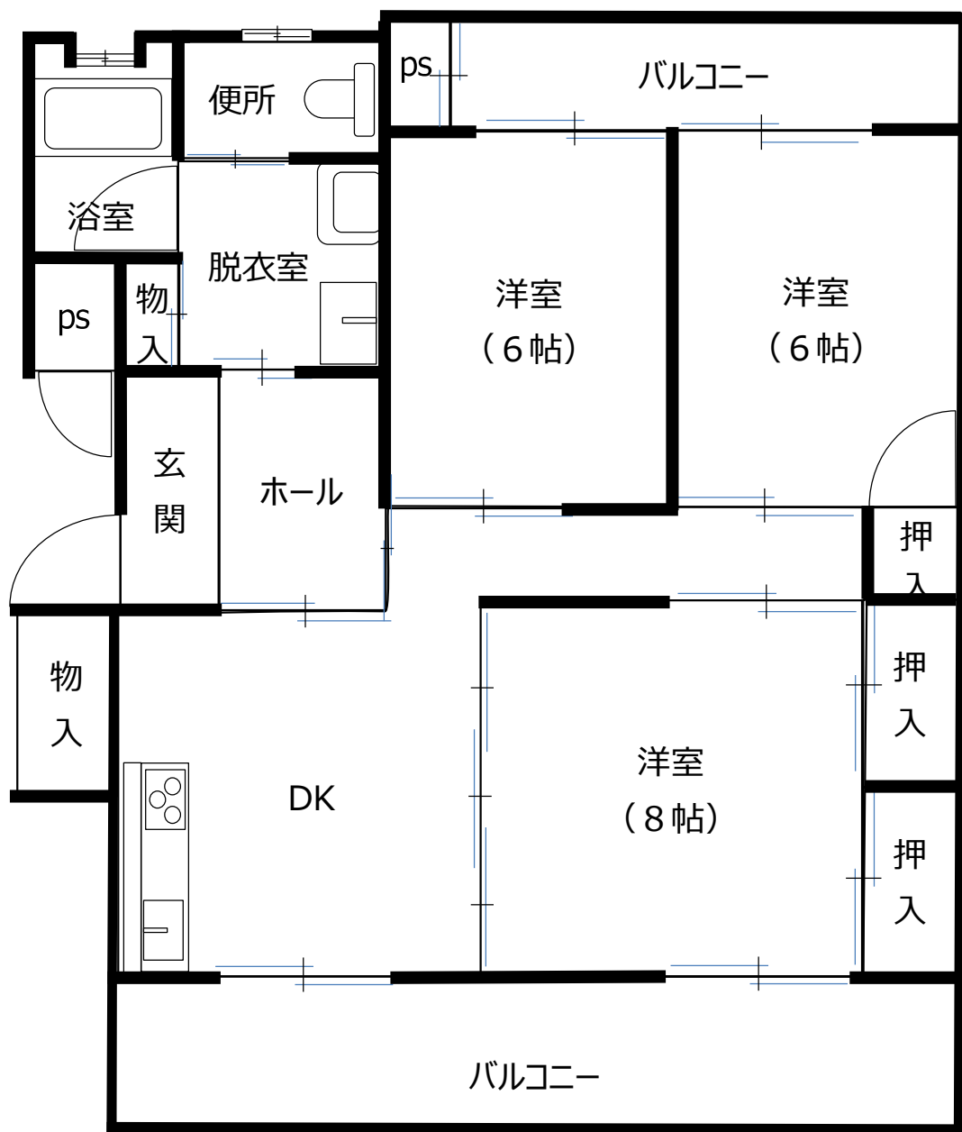
【 八雲住宅3DK 間取り 】
