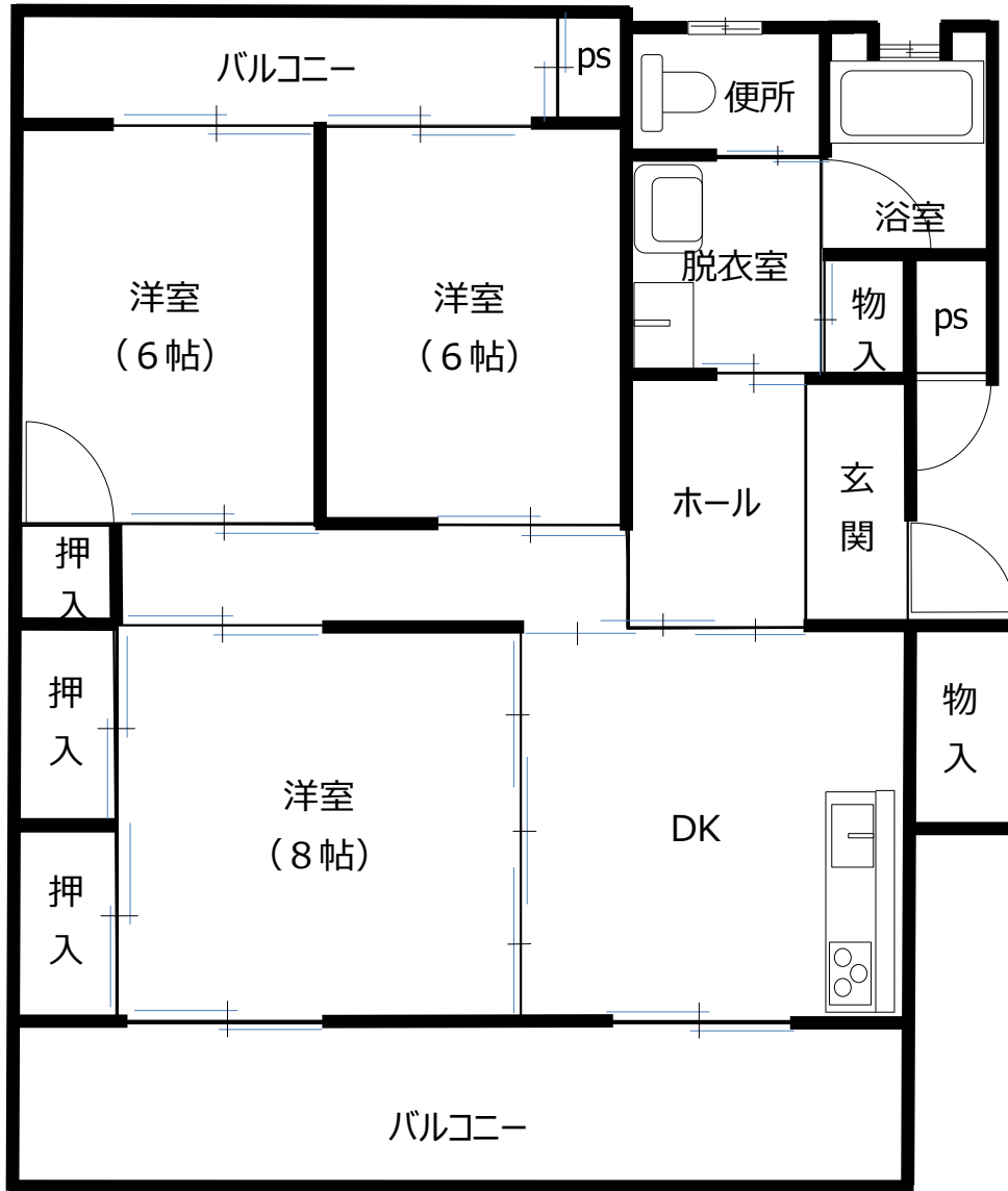
【 八雲住宅3DK 間取り 】
