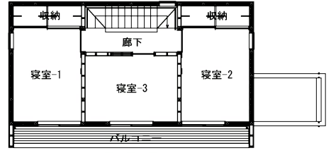
2階平面図
