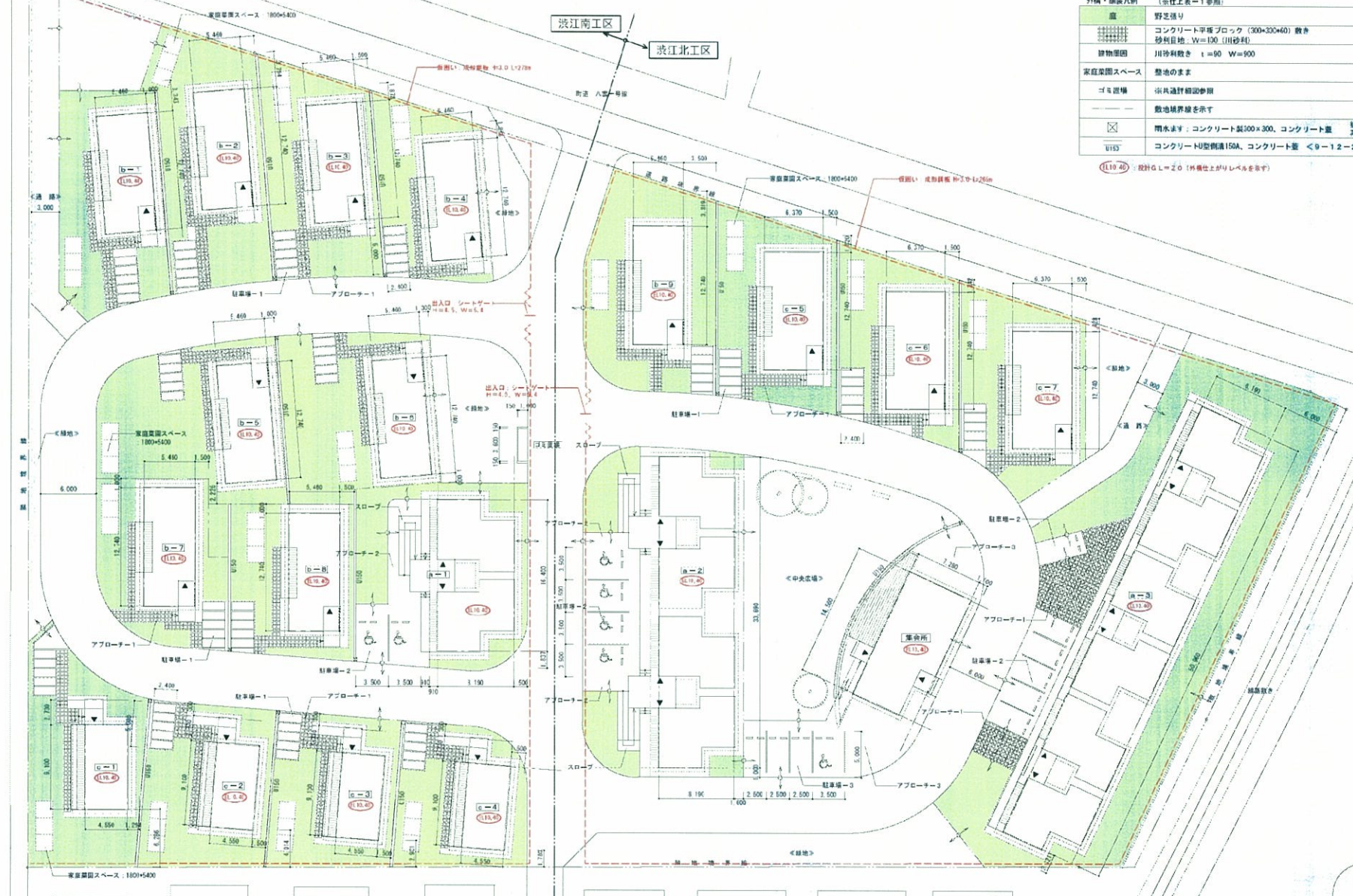
洗江地区 配器図
